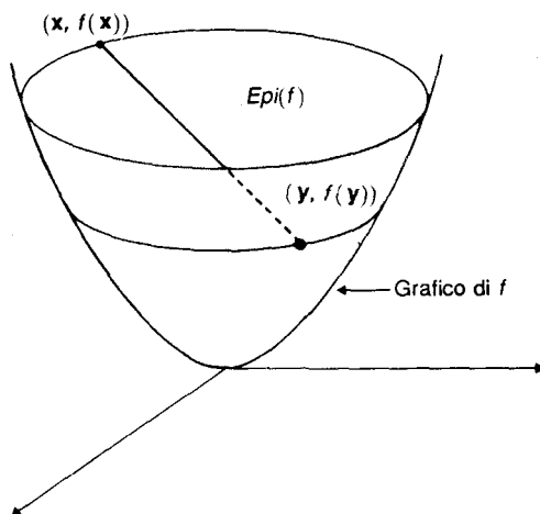
Fig. 7.6 Funzione strettamente convessa.
