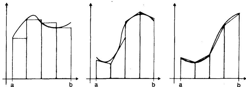
Fig. 8.4 a) Metodo dei rettangoli
