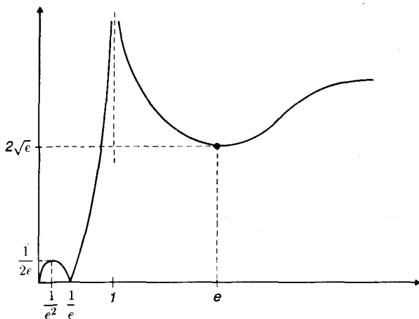
Fig. 6.29 Grafico qualitativo di y = \sqrt{x} \left| 1 + \frac{1}{\log x} \right| .
