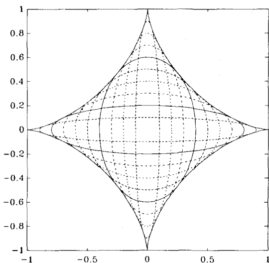
Fig. 7.29 Astroide come involuppo di ellissi.
